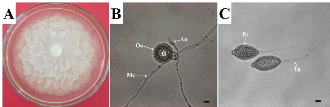
Figura 1. Características de Phytophthora capsici . A) Crecimiento del oomiceto sobre una caja de Petri conteniendo medio de cultivo. B) Micelio cenocítico (Mc), y anteridio (An); gametangio masculino (Oo); gametangio femenino (O) y oospora (O; espora sexual). C) Esporangio (Es) produciendo tubo germinativo (Tg). Barras (A-B): 10 µm. (Imágenes cedidas por Ailton Reis).
