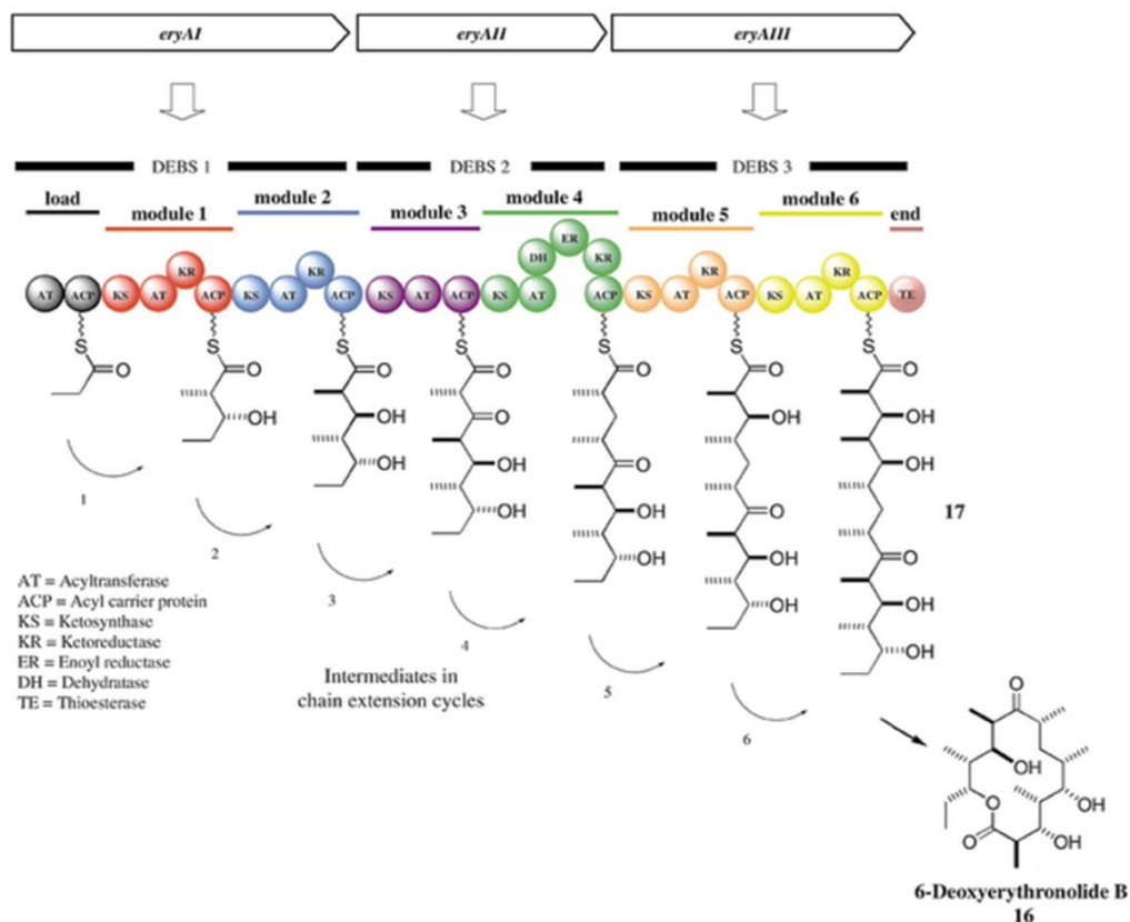
Figura 9. Biosíntesis de macrólidos vía acetato.
