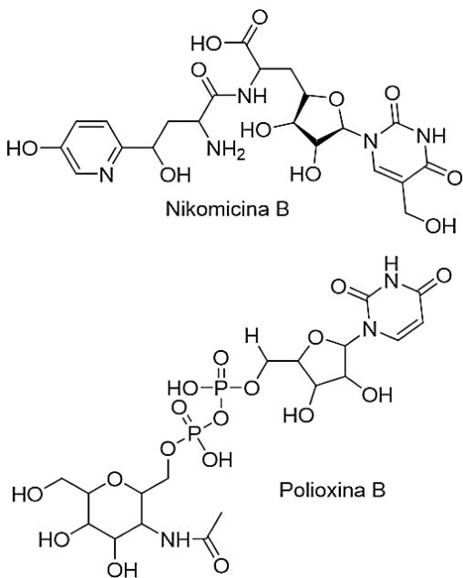
Figura 5. Péptidos nucleósidos Nikomicina B y Polioxina B.
