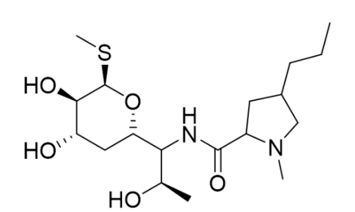
Figura 6. Nuevo agente antifúngico: Cifomicina.
