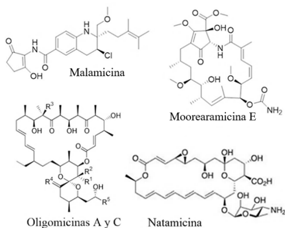
Figura 7. Metabolitos y antibióticos producidos por actinobacterias con actividad antagonista contra un amplio espectro de patógenos.
