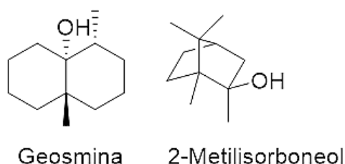
Figura 1. Compuestos orgánicos volátiles (COV): Geosmina y 2-metilisorboneol.
