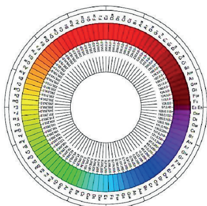
Figura 1. Óptica Pura y Aplicada Fuente: Color y Música: Relaciones Físicas entre Tonos de Color y Notas Musicales. (Perez y Gilabert, 2010).
