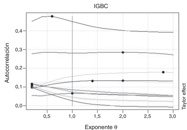
Figura 9. Autocorrelación de los retornos absolutos para diferentes \theta para los primeros 10 rezagos ( k = 1... 10 ). Cálculos propios.
