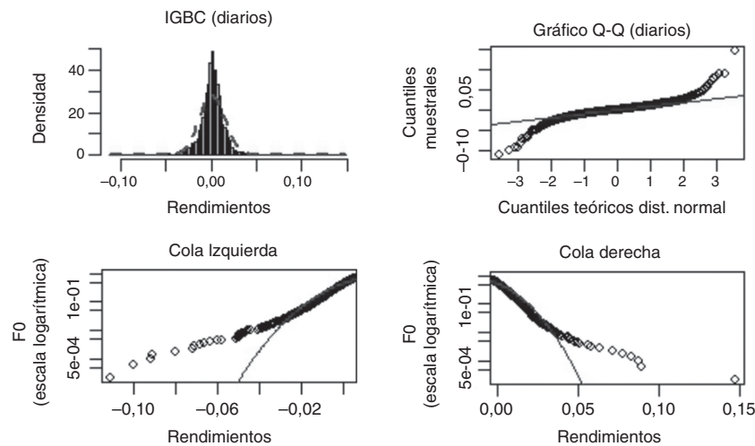
Figura 5. Histograma, QQ-plot, cola izquierda y cola derecha de los rendimientos de IGBC.
