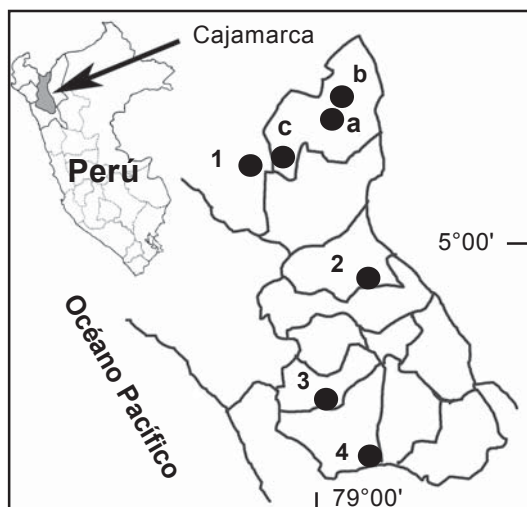
Figura 1. Distribución de las Podocarpaceas en los bosques montañosos del norte del Perú. (1) Canchaque, (2) Cutervo, (3) Tongod, (4) Cachel, (a, b, c) San Ignacio.
