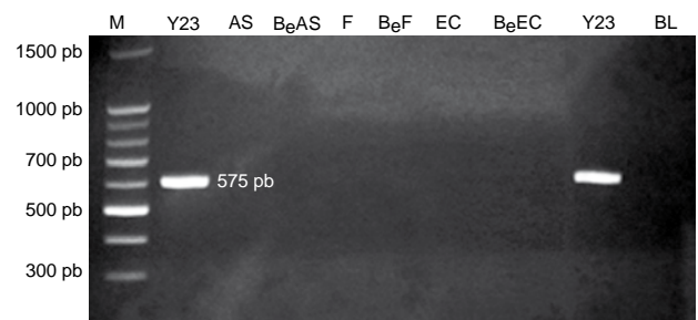
Figura 3. M: Ladder, Y23: Yersinia ruckeri (control positivo), AS: Aeromonas salmonicida , BeAS: Blanco de extracción (Kit) para A. salmonicida , F: Flavobacterium sp., BeF: Blanco de extracción (Kit) para Flavobacterium sp., EC: Escherichia coli , BeEC: Blanco de extracción (kit) para E. coli , BL: Blanco de PCR.
