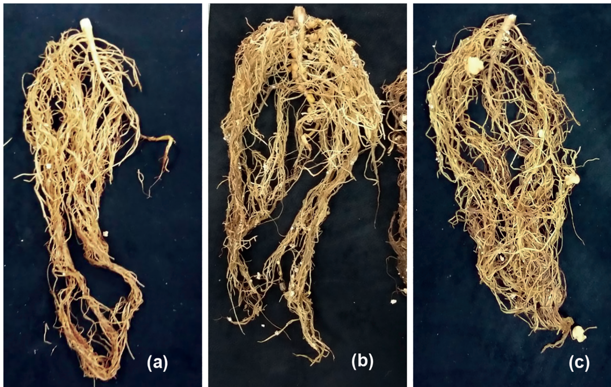
Figura 1. Distribución de los nódulos en las raíces de Lupinus mutabilis . A. Sin presencia de nódulos; B. Presencia de nódulos en las raíces principales y secundarias; C. Nódulos solo en raíces secundarias.
