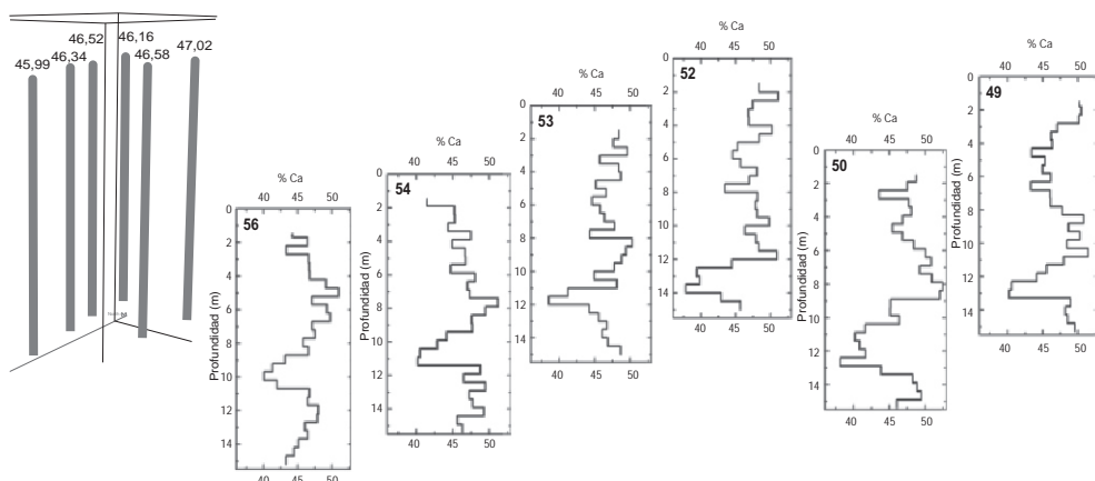
Figura 9. Perfil de las concentraciones de CaO en las perforaciones de voladura del proyecto 2720 de la cantera de Atocongo en función de la profundidad.
