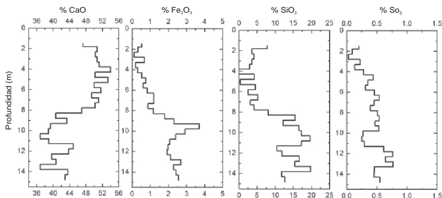
Figura 8. Perfil de concentraciones de CaO, Fe 2 O 3 , SiO 2 y SO 3 en la perforación de voladura 232 de la cantera de Atocongo en función de la profundidad.
