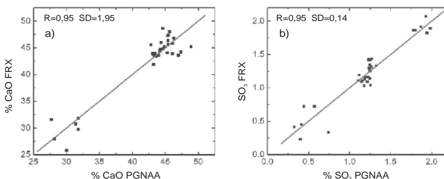
Figura 5. Correlación de las concentraciones de (a) CaO y (b) SO 3 obtenidos por FRX y calculados por PGNAA.
