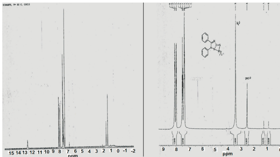
Figura 3. Espectros RMN- H^1 del ligando a 60°C (izquierda) y del complejo de plomo (derecha)
