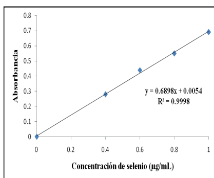
Figura 3. Curva estándar de Se(IV) a 570 nm en presencia de medio YEPD estéril.
