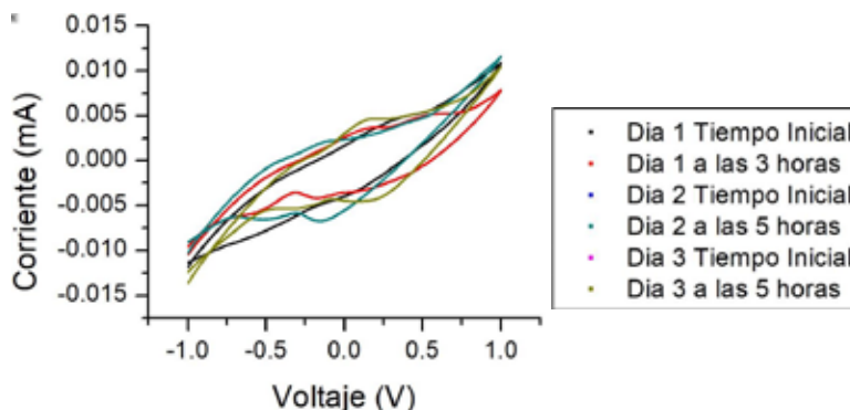
Figura 4. Voltametría Cíclica del sustrato inoculado con el cultivo de At. ferrooxidans (cepa 151).
